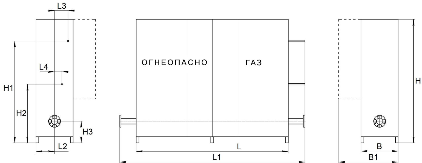
Рисунок П.1 – Габаритные размеры ПУГ
